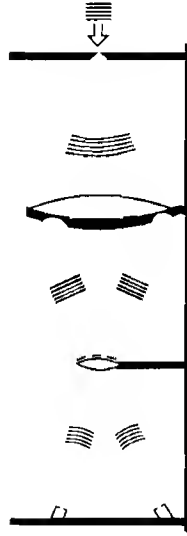
شكل ٩-٢٥: تجربة ويلر للشق الطولي المزدوج، والاختيار المتأخر.
